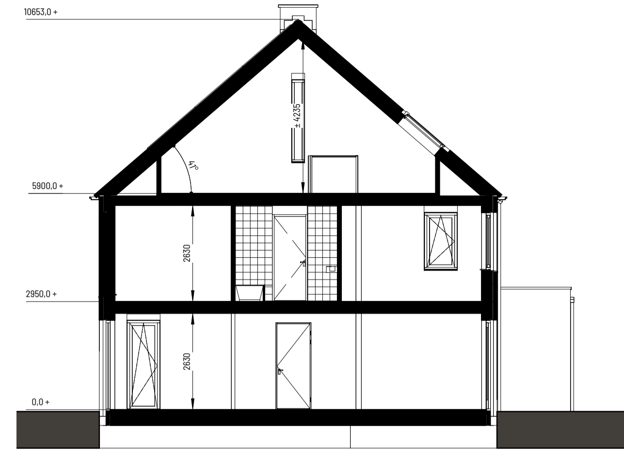
doorsnede 1:100
