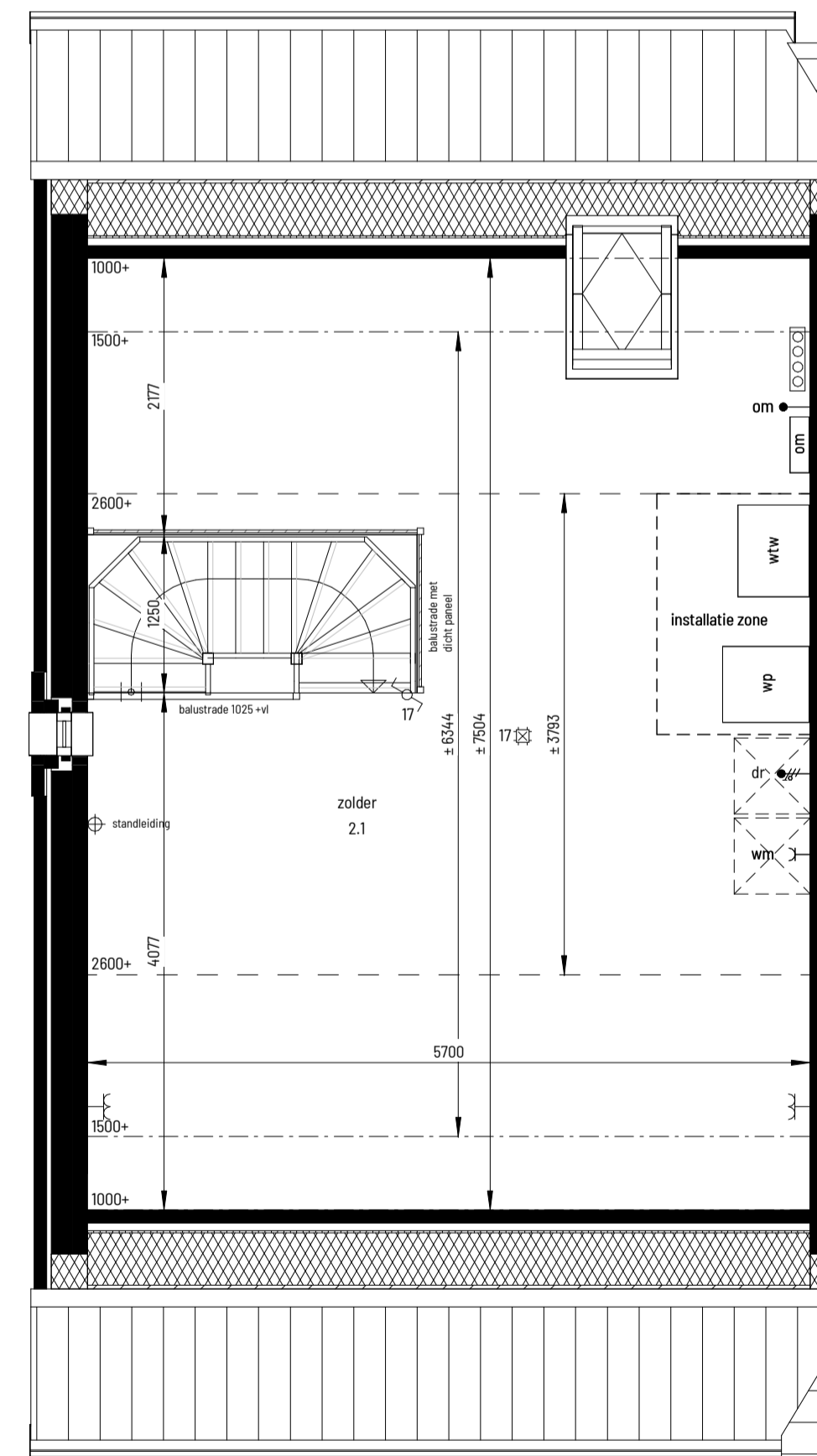
tweede verdieping 1:50
